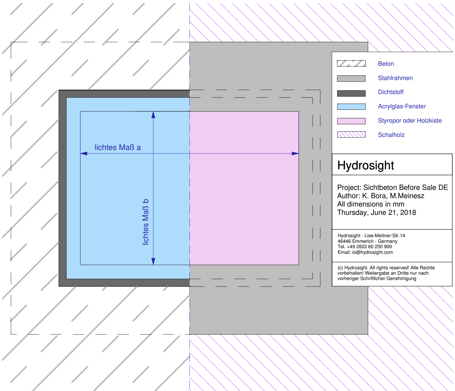
Querschnitt nach Fertigstellung
