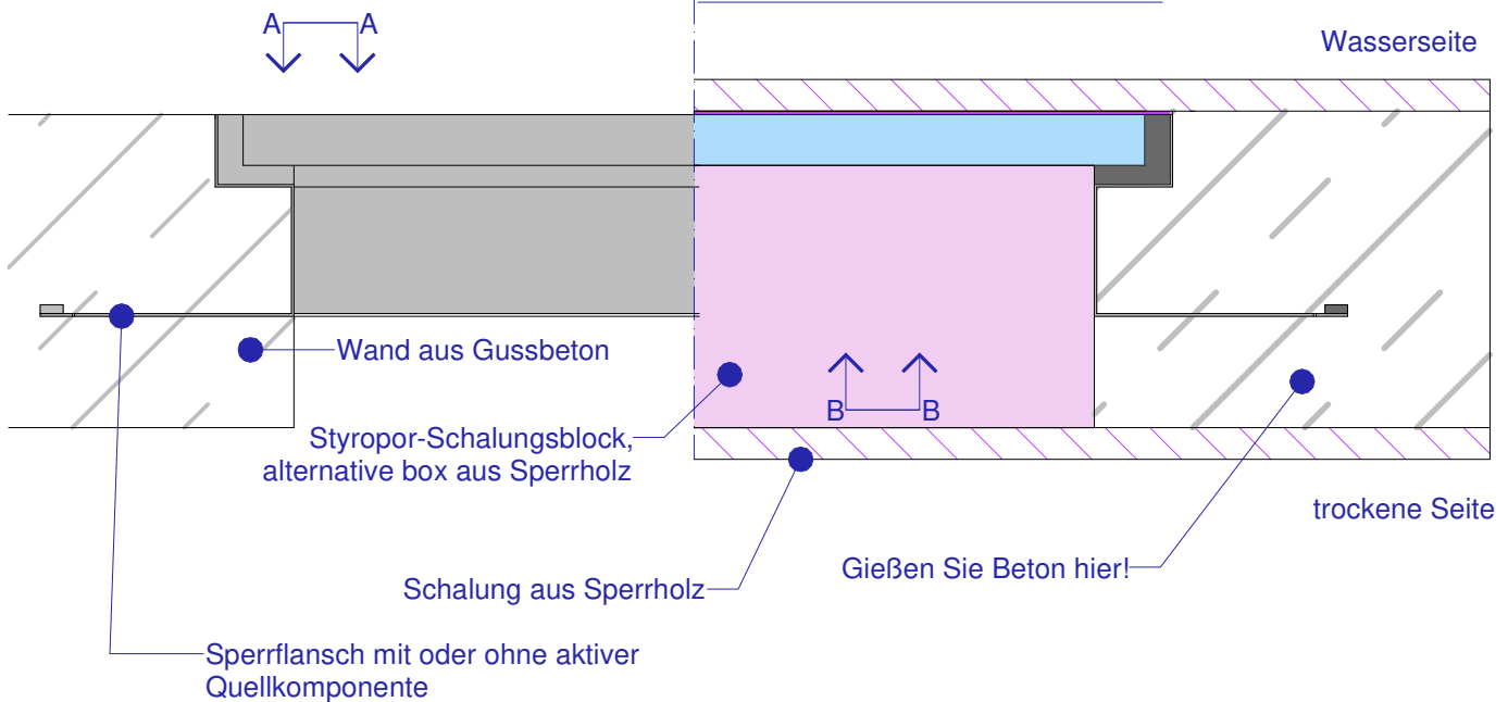
Querschnitt nach Fertigstellung
